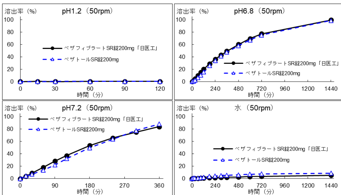
(溶出曲線)
