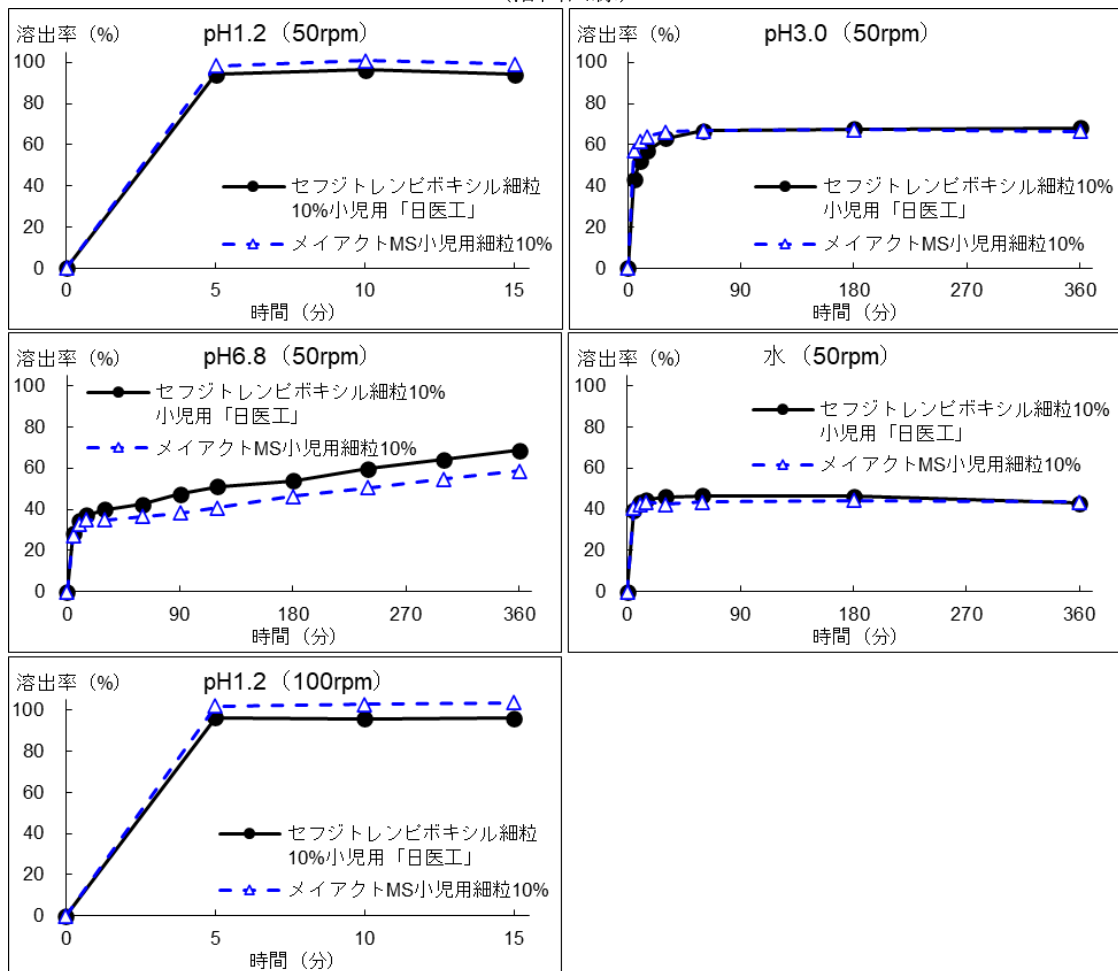
(溶出曲線)
