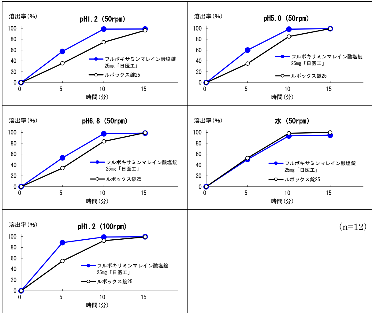
(溶出曲線)
