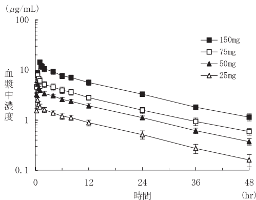
薬物動態学的パラメータ
