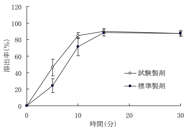
<pH6.8、50rpm>
